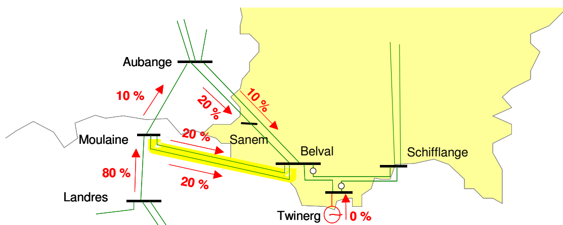
Bild .3: Belastung der Kuppelleitungen von Sotel bei Starklast nach Neubau einer 220- kV-Doppelleitung Belval \leftrightarrow Moulaine
