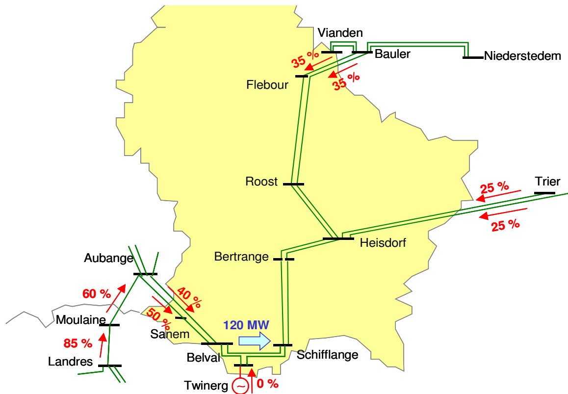
Bild .5: Leistungsfluss-Verschiebung von 120 MW über Luxemburg bei Zusammenschaltung der Netze von Cegedel und Sotel
