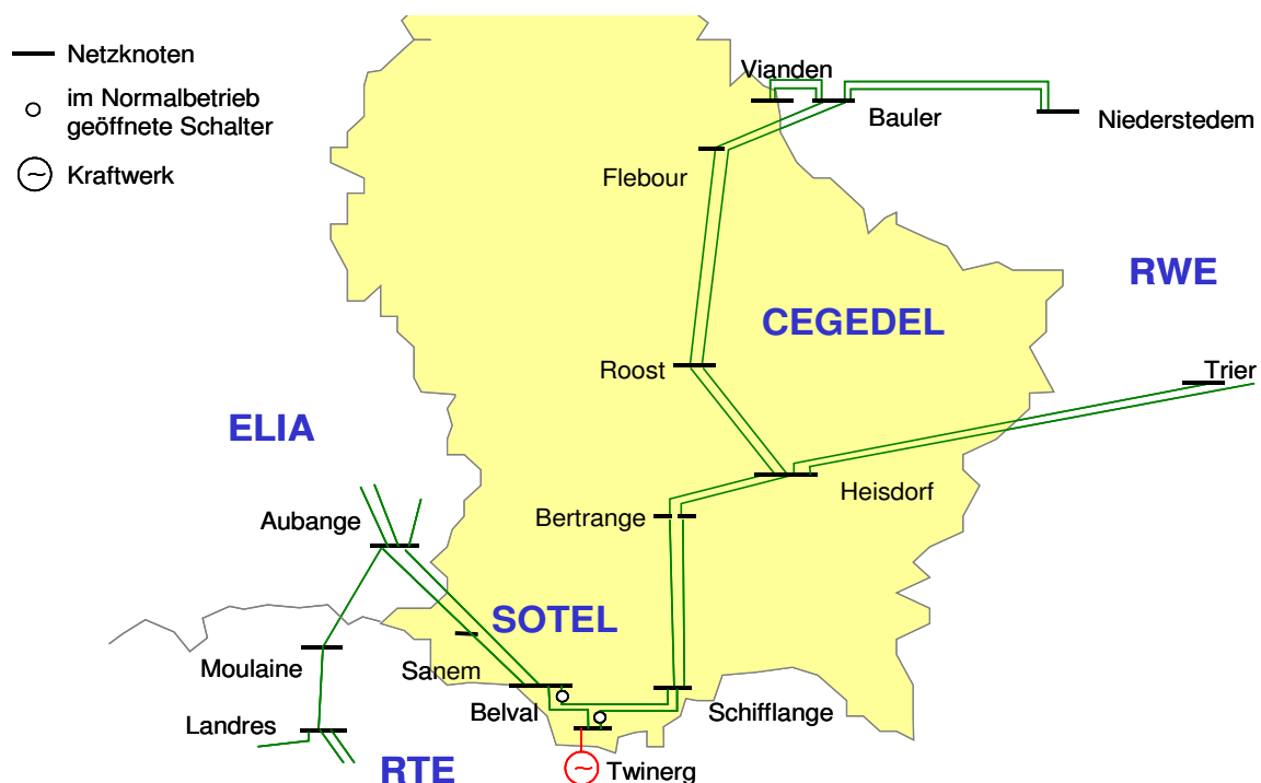
Bild .1: Schematischer Plan der 220-kV-Netze im Ist-Zustand (Sotel- und Cegedel-Netze getrennt)
