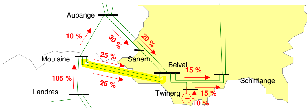
Bild .6: Belastung der Leitungen bei Zusammenschaltung der Netze von Cegedel und Sotel und Zubau der 220-kV-Doppelleitung Belval↔Moulaine
