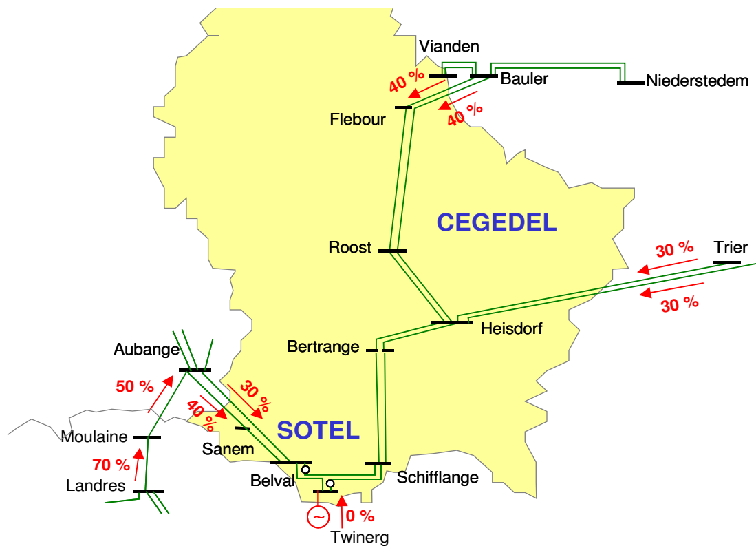
Bild .2: Netzbelastung im Ist-Zustand bei Starklast (Sotel- und Cegedel-Netze getrennt)
