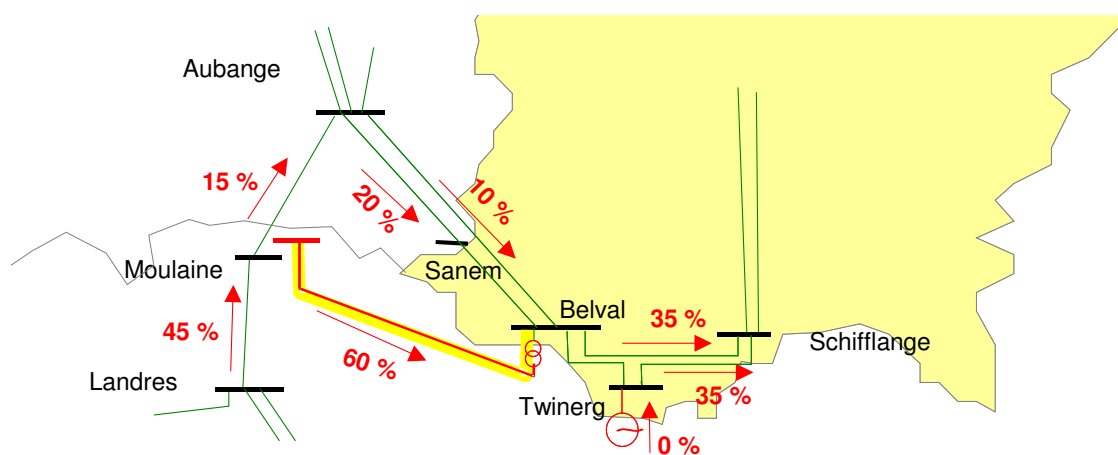
Bild .8: Belastung der Leitungen bei Zusammenschaltung der Netze von Cegedel und Sotel und Zubau einer 380-kV-Einfachleitung Belval ↔ Moulaine
