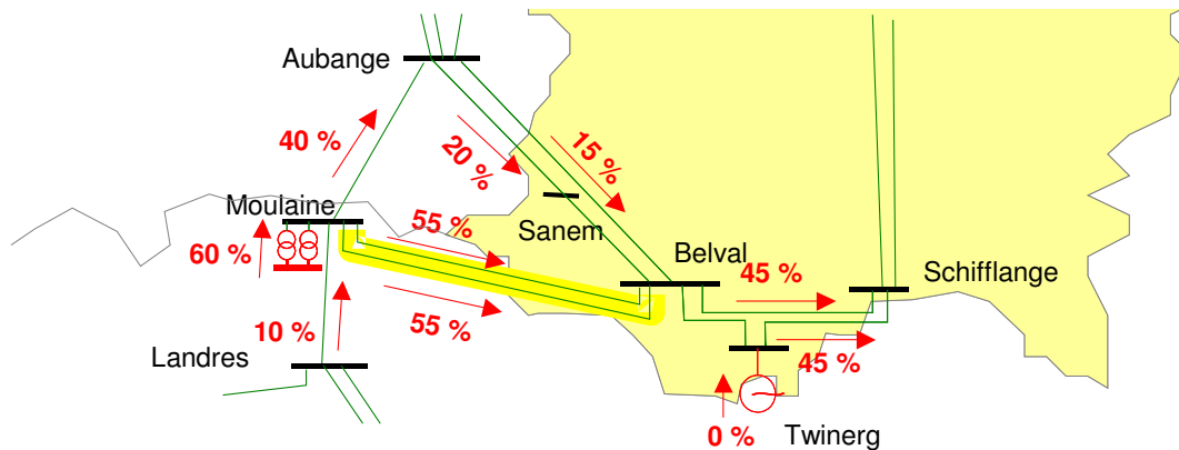
Bild .7: Belastung der Leitungen bei der hier betrachteten Netzvariante nach der Errichtung zweier 380/220-kV-Transformatoren in Moulaine
