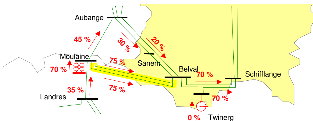
Bild .4: Belastung der Leitungen bei komplettem Wegfall der Versorgung aus dem RWE-Netz unter Annahme der Errichtung zweier Netzkuppeltransformatoren in Moulaine
